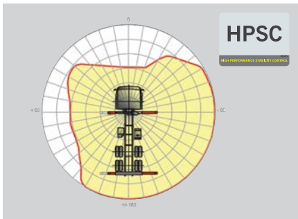
HPSC Monitoramento simultâneo de estabilidade e capacidade de carga
